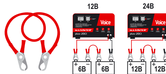
Рисунок 3. Соединительный кабель с зажимами для одновременной последовательной зарядки двух АКБ (в комплекте)
